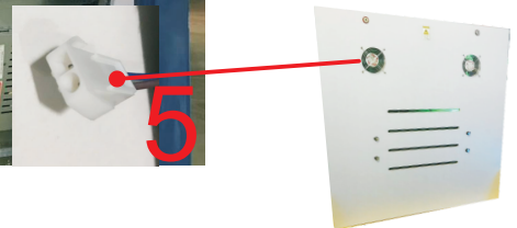
Connect fan wire harness
